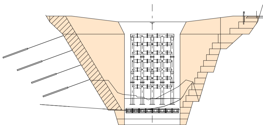
水沢第3砂防堰堤を下流から見た図
