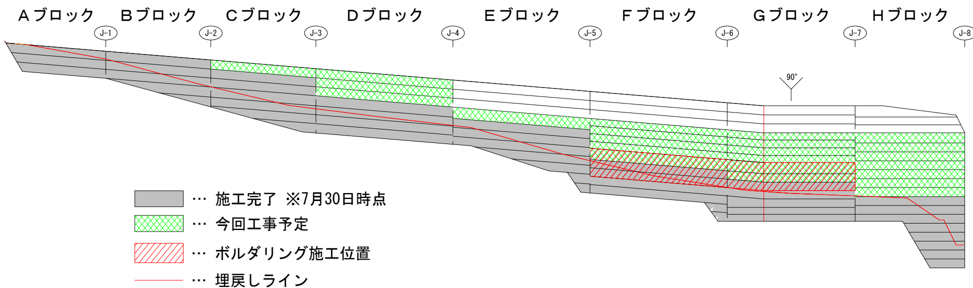
堰堤正面図
