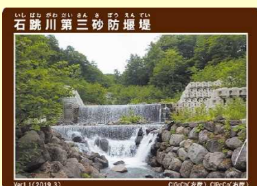
石跳川第三砂防堰堤 (いしばねがわだいさんさぼうえんてい)
