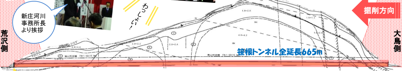
笹根トンネル縦断面図
