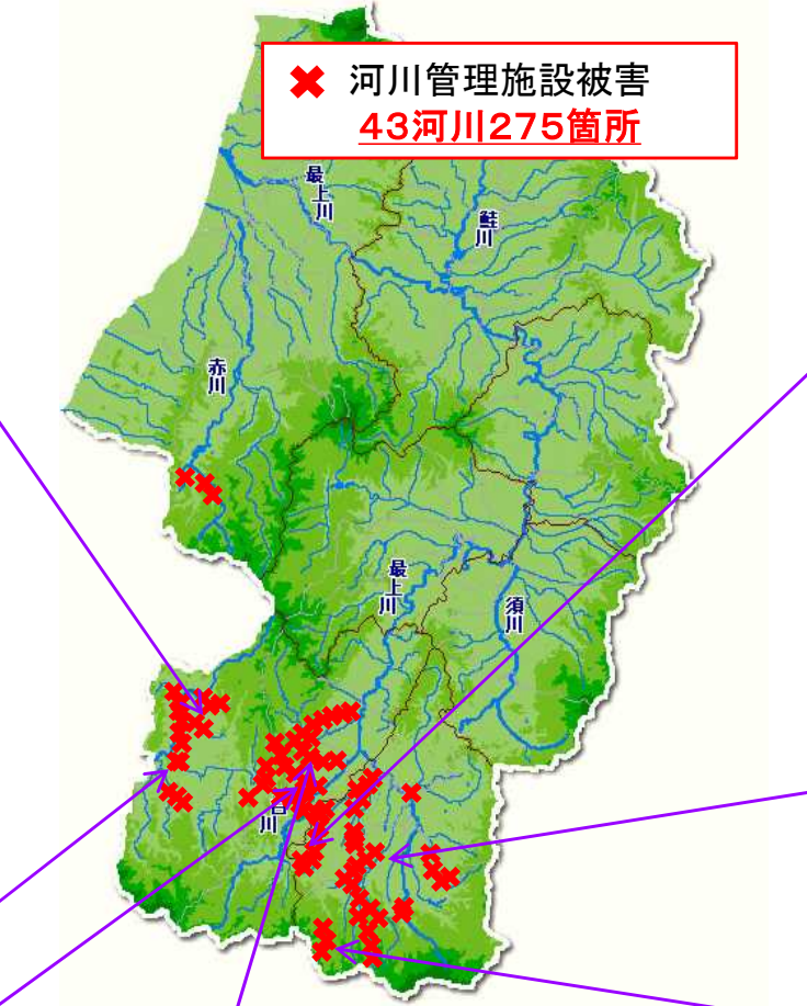
広範囲に渡る護岸損壊・土砂堆積・浸水
