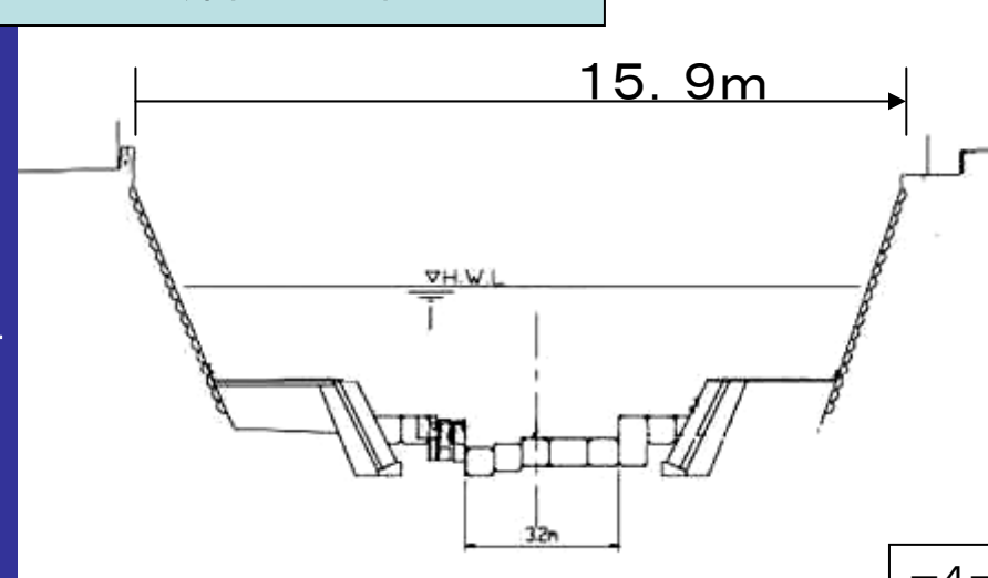
横断図 (西灘橋付近(国道2号))
