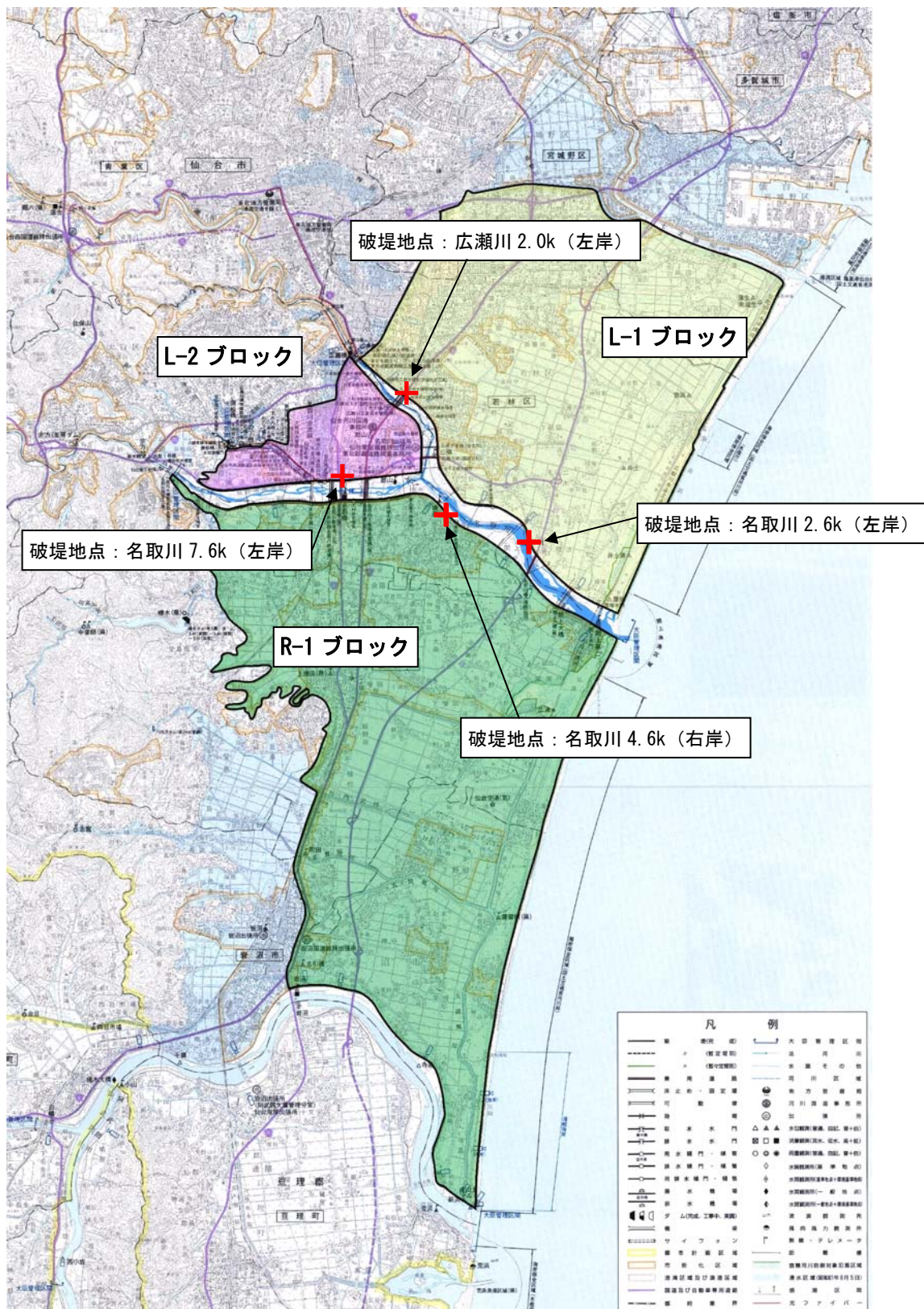
様式-1 氾濫ブロック分割図 名取川・広瀬川
