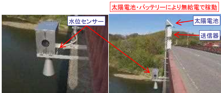
危機管理型水位計設置状況（郡山市西田町鬼生田地先（阿武隈川））
