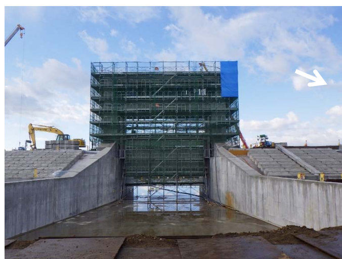
上屋・ゲート施工状況（H29.2.6撮影）
