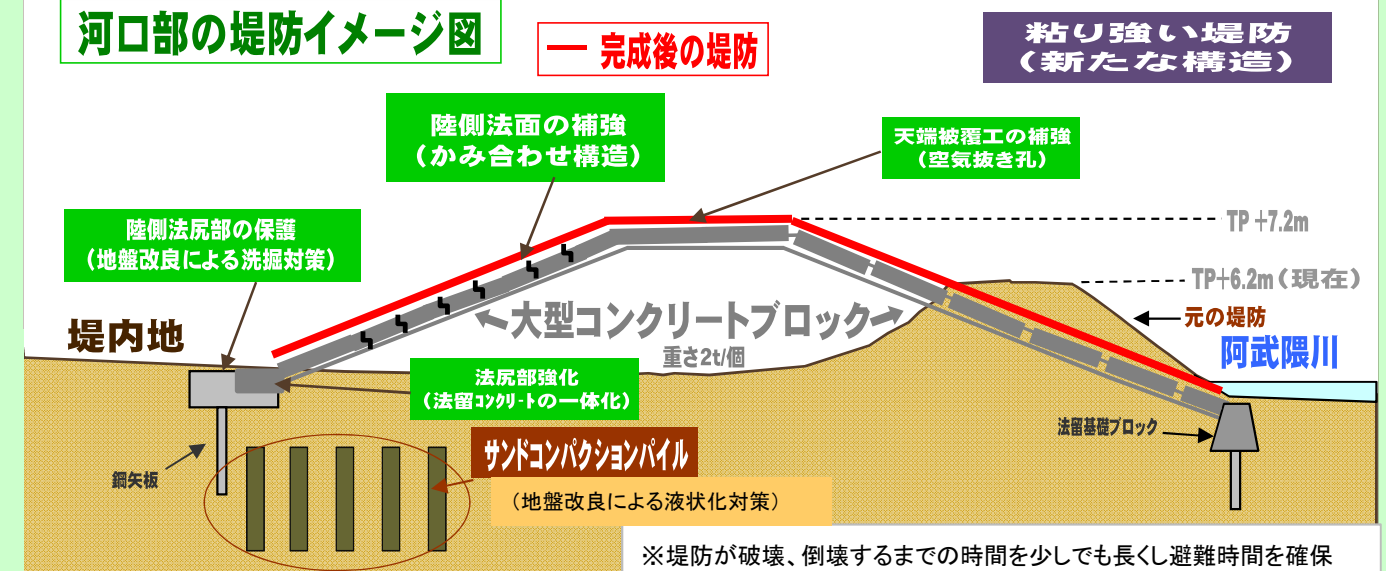
阿武隈川下流荒浜5工区堤防災害復旧工事
