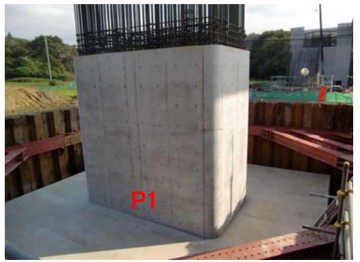
③ 高松橋 橋脚(P1)
