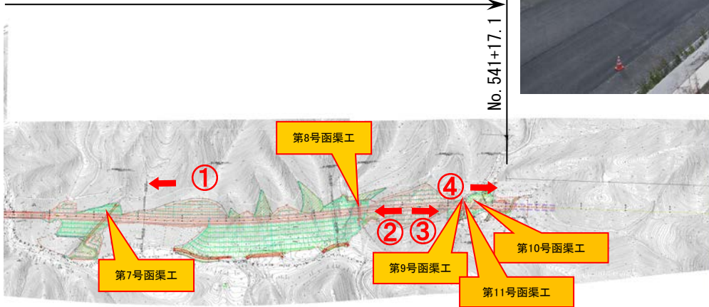
朝田貴地区舗装工事 受注者：前田道路(株) 工期：H27.4.1～H28.3.18
