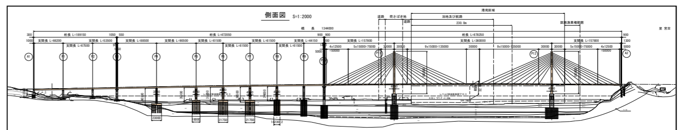
(仮)気仙沼湾横断橋 全体一般図
