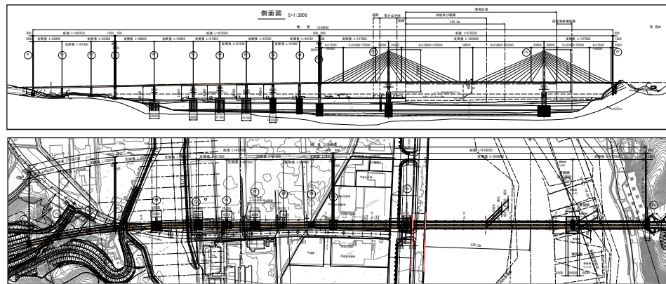
気仙沼湾横断橋(仮)全体一般図
