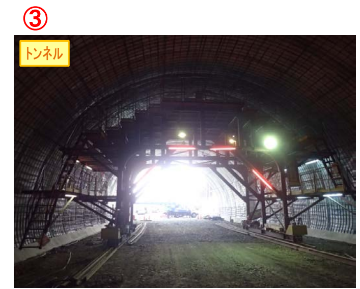
③ ▲唐桑トンネル(仮)坑内(覆工の様子)
