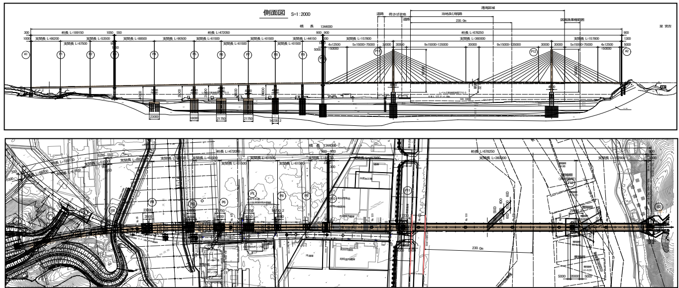
気仙沼湾横断橋全体一般図
