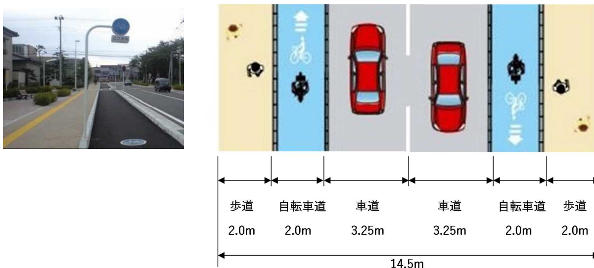
写真・図 自転車道整備例
