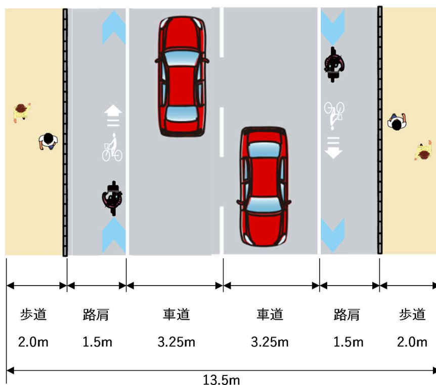
写真・図 自動車交通量が 10,000 台/日以上 of 郊外部 ( DID 地区以外 ) の幹線道路での整備例 図出典：国ガイドラインをもとに作成
