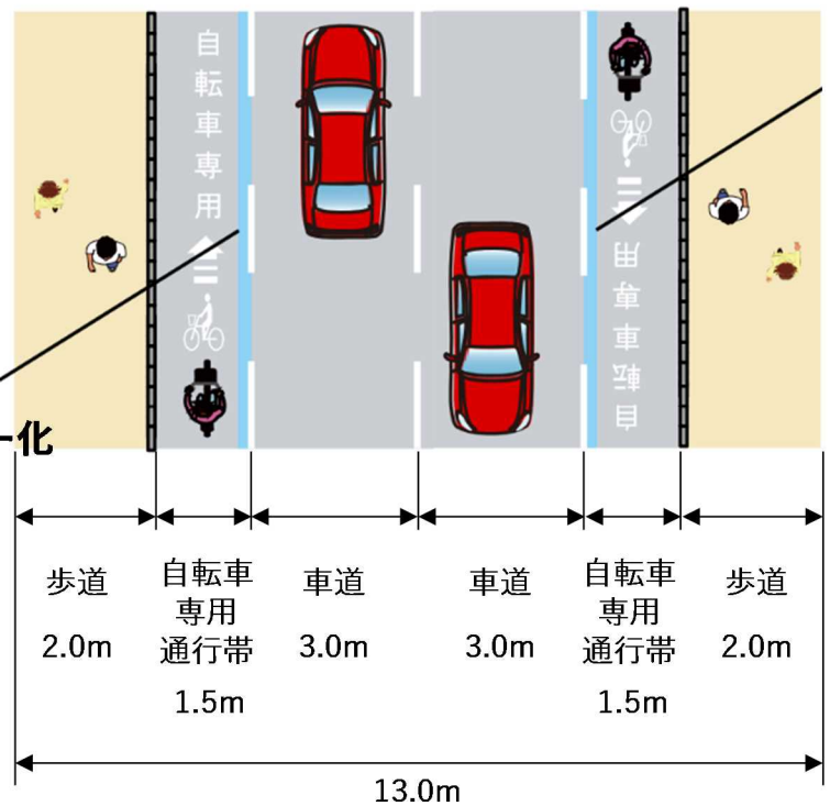
写真・図 自動車交通量が 10,000 台/日以上 の DID 地区の幹線道路での整備例
