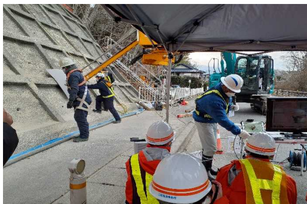
▲無線で操作できるバックホウドリル
