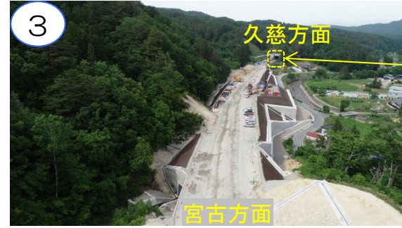
萩牛トンネルと電気室の工事中です。
