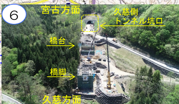
萩牛トンネルと普代川大橋の橋台・橋脚を工事中です。
