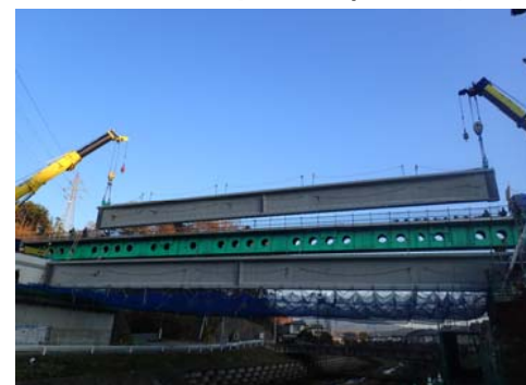
架設中(クレーン2台で相吊)
