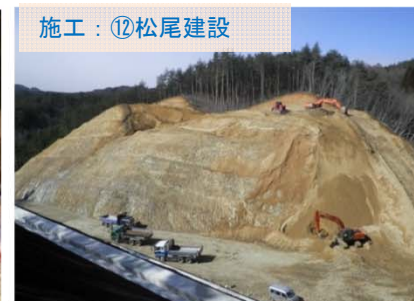
施工：⑫松尾建設 山をけずって、土を搬出しています。道路が更に広くなります。
