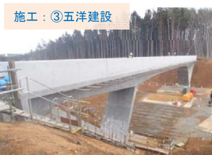
施工：③五洋建設 青野滝地区の、道路の上をまたぐ橋（跨道橋：こどうきょう）が、ほぼ出来上がりました。
