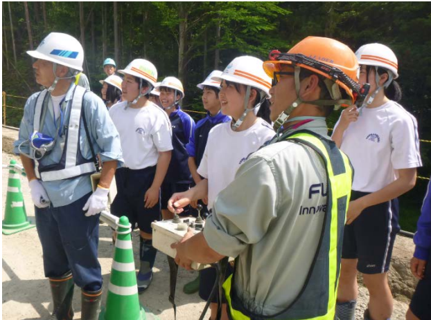
▲トンネルの内壁にコンクリートを吹き付ける大型機械の遠隔操作をいざ体験！
