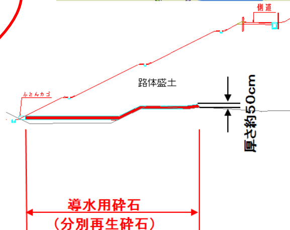
▲導水工側面図
