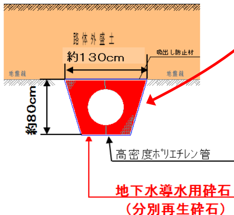
▲地下排水工断面図
