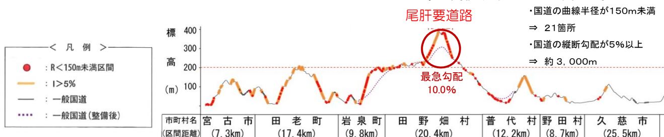
▲国道45号(宮古市～久慈市)の線形不良箇所の状況
