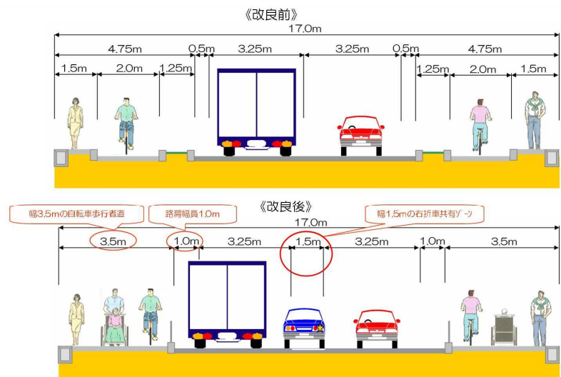
断面図
