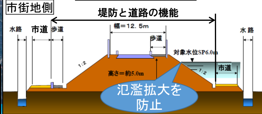
二線堤 標準断面図
