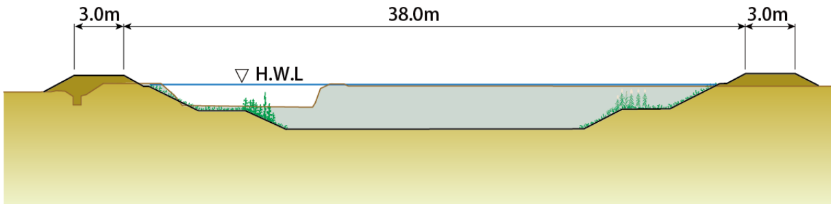
目標流量18m 3 /s区間の標準断面図
