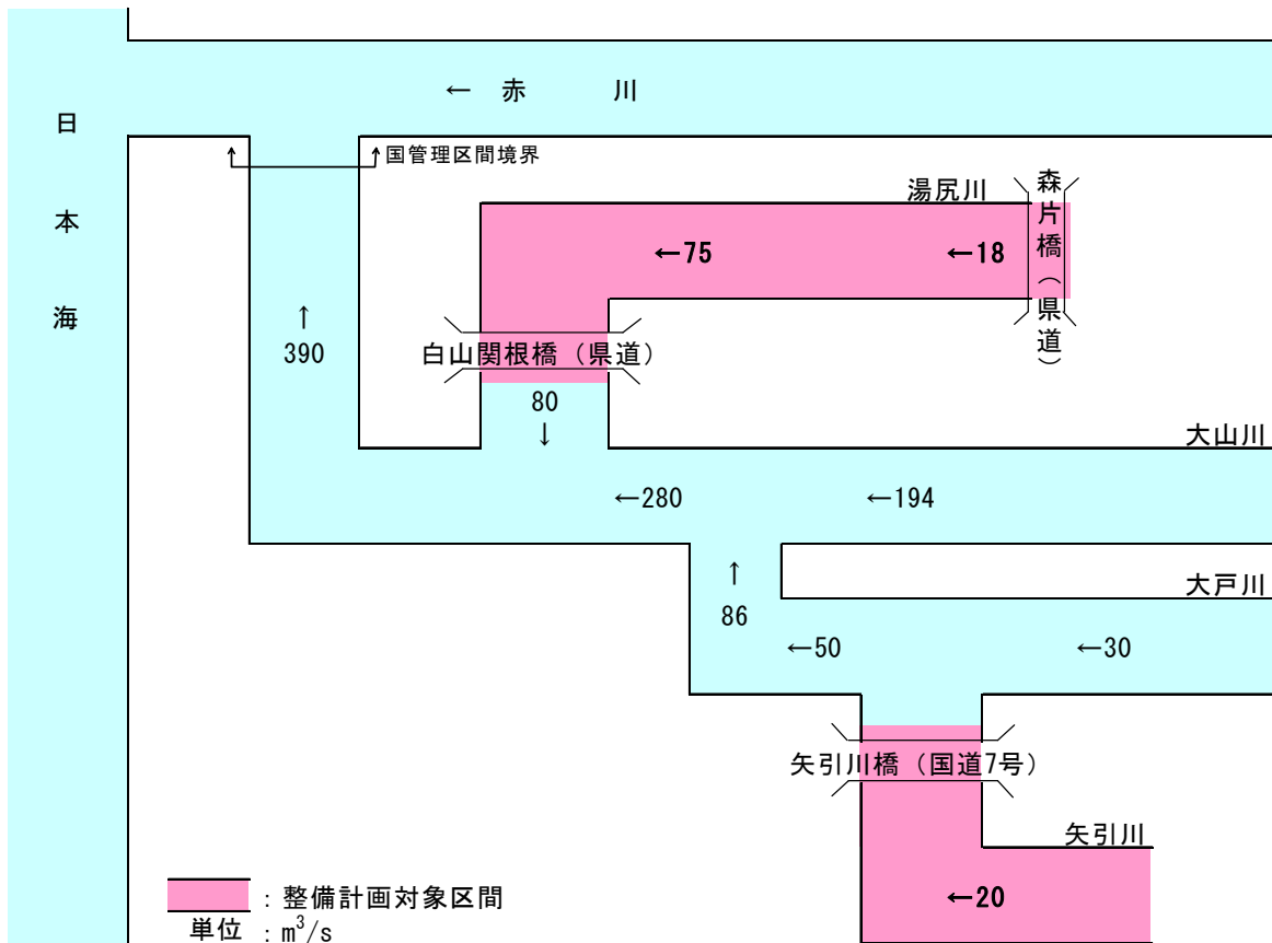
<主要地点における河道の配分流量>
