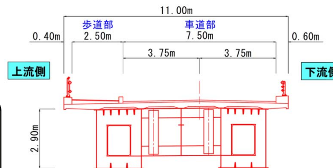
▲ 橋梁断面図
