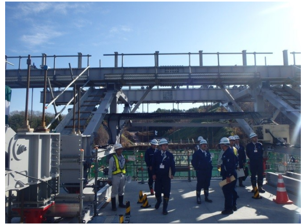
▲「青の滝川橋」上部工桁架設状況の見学
