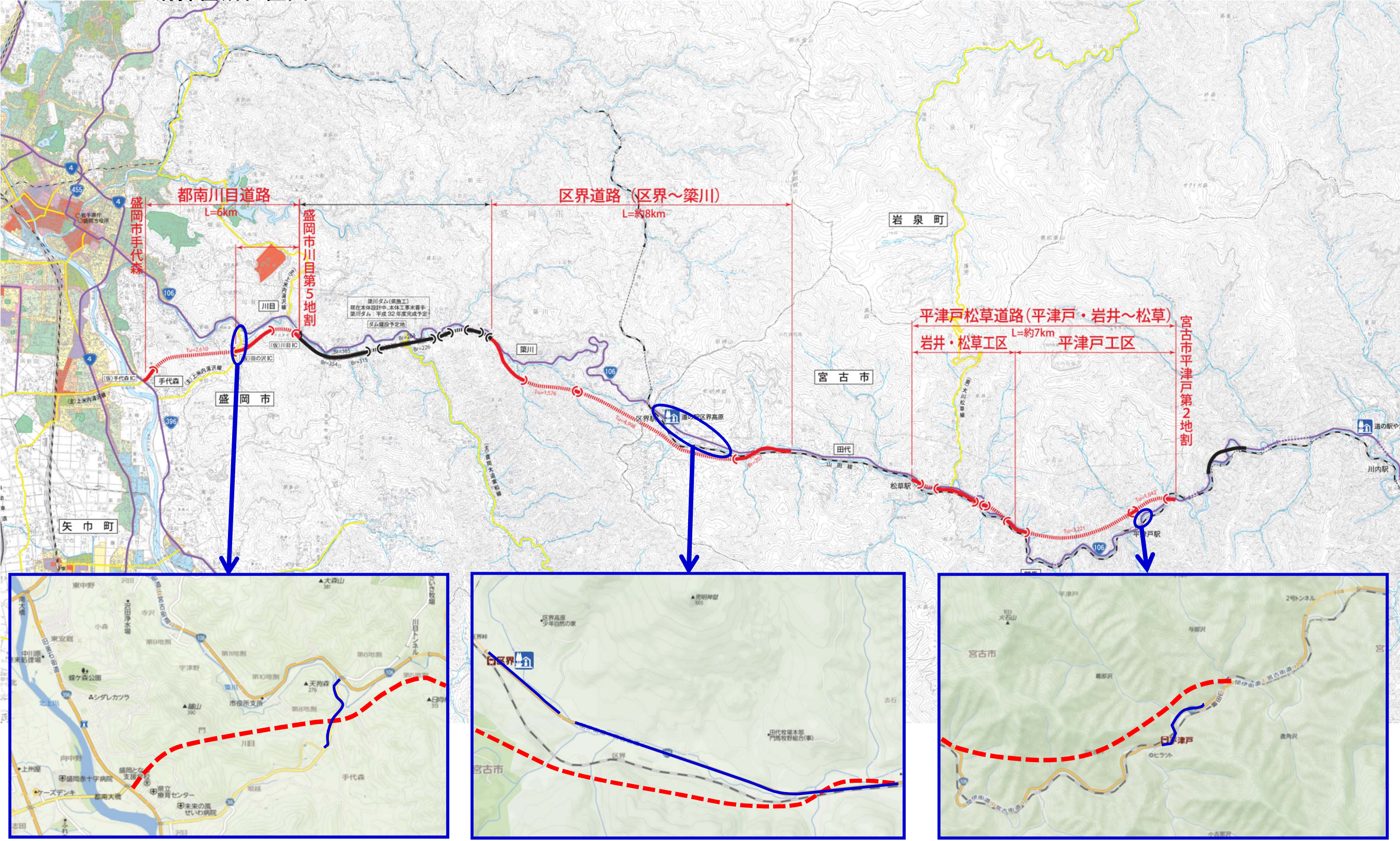
手代森地区:上米内湯沢線 手代森トンネル出入り口前後50m区間
