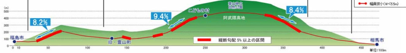
【縦断面図】
