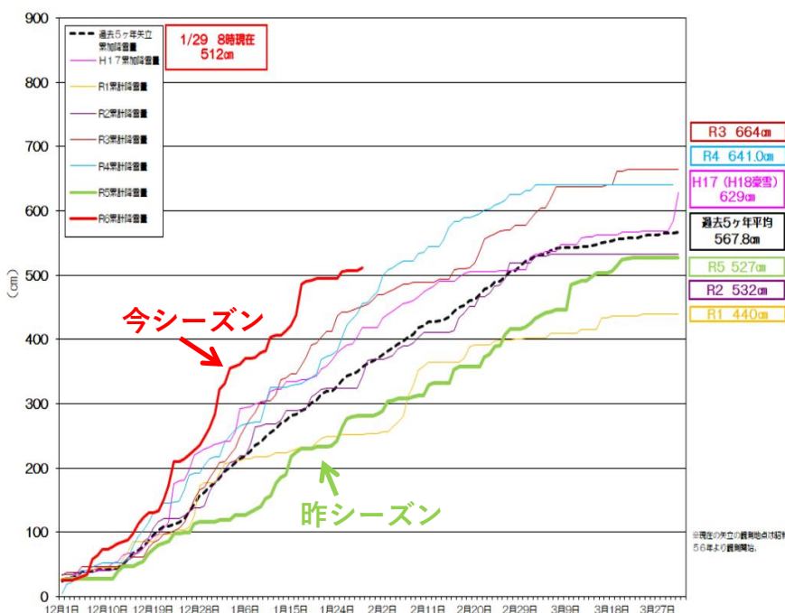
令和6年度 能代管内降雪データ 累加降雪量(矢立)
