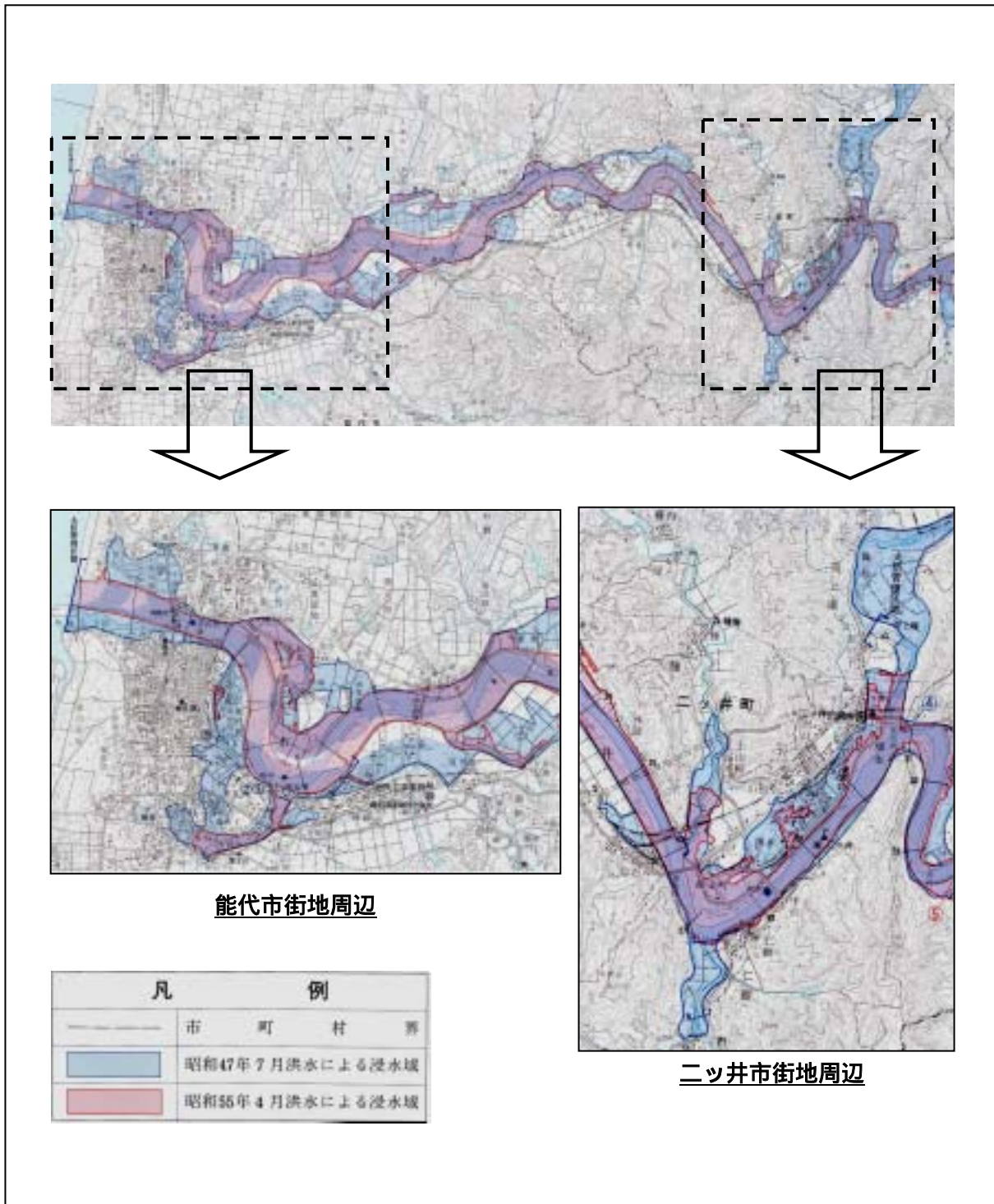
図2 - 8 昭和47年7月, 昭和55年4月洪水浸水実績図
