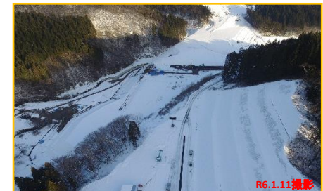
【大型函渠部】 路体盛土工 4段目まで完了
