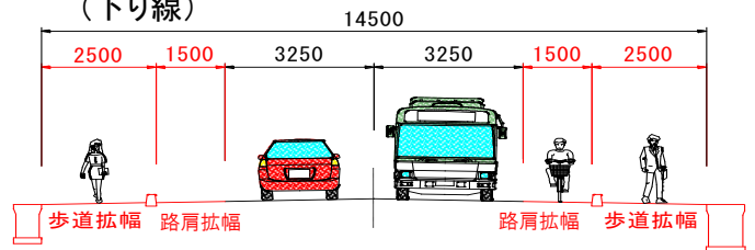
《計画横断面》 (下り線)
