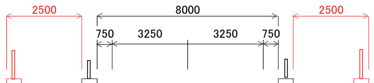
【計画横断面】
