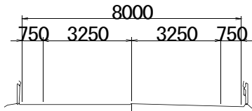
【現況横断面】
