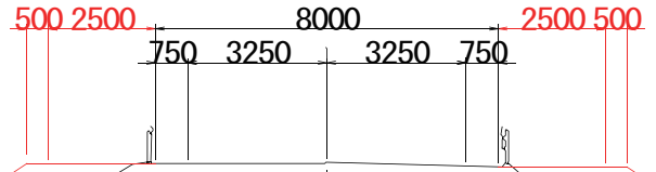
【計画横断面】
