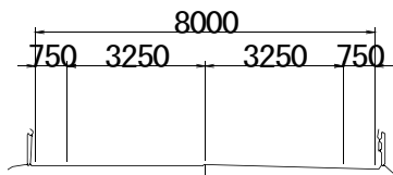
【現況横断面図】
