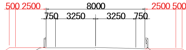
【計画横断面図】
