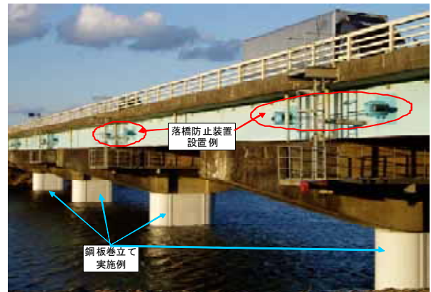
▲耐震補強の実施例
