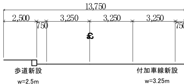
▲ 計画横断面図
