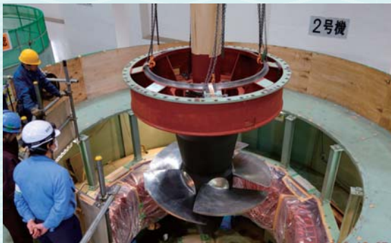
水車ランナ吊り込み作業中
