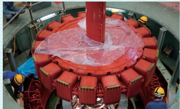
発電機(回転子)吊り出し作業中
