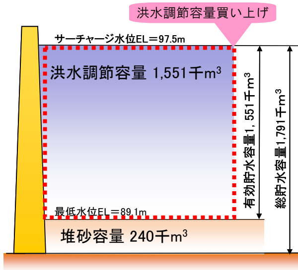
図 小羽広ダム 容量配分図
