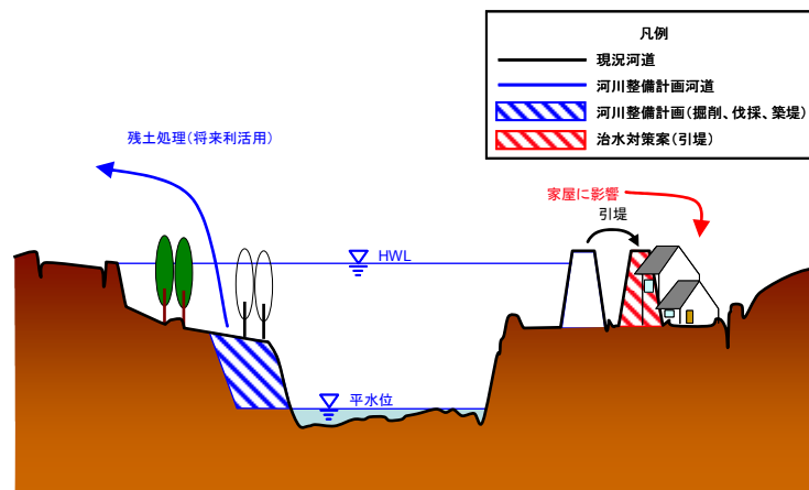
図 4.2-45 河川改修イメージ（ケース 4）
