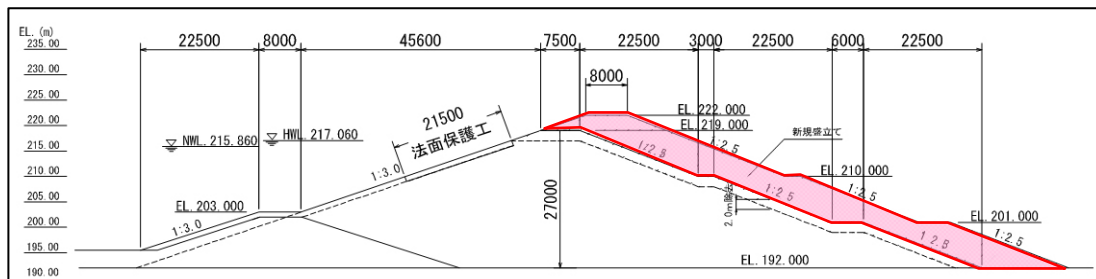
図 八塩ため池 かさ上げイメージ
