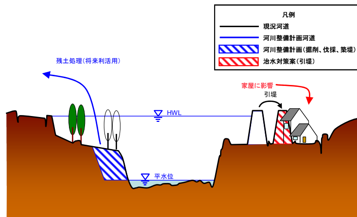
図 4.2-45 河川改修イメージ（ケース 4）
