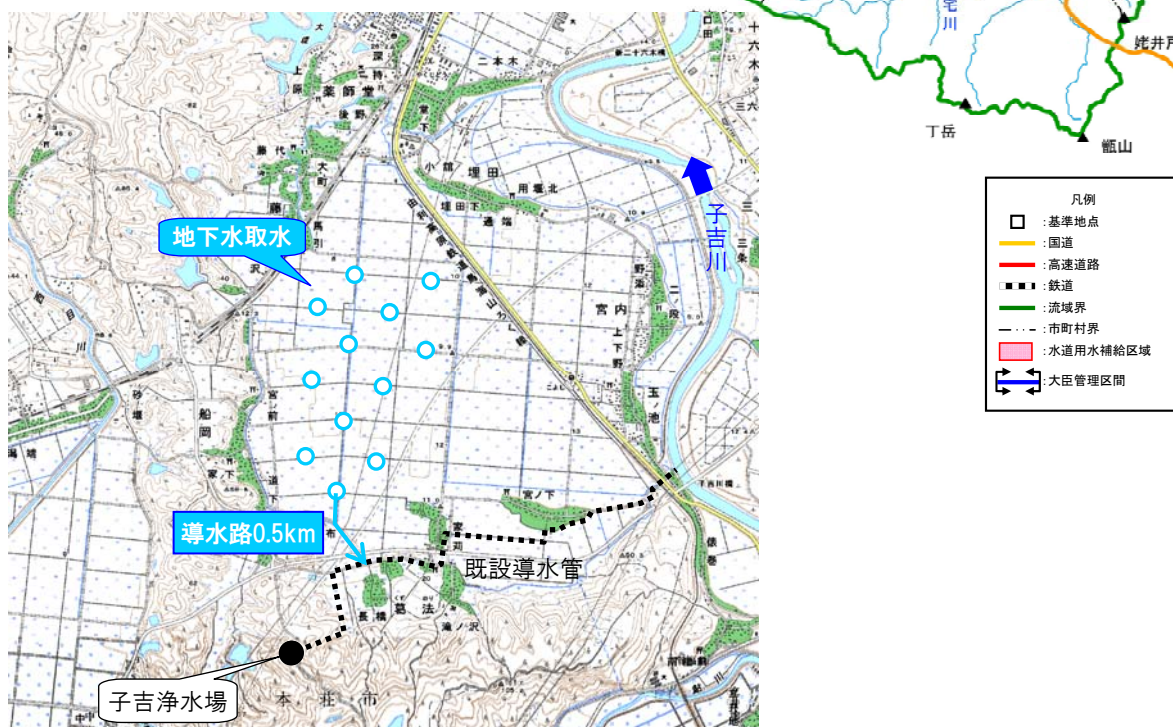
図 揚水井配置図
