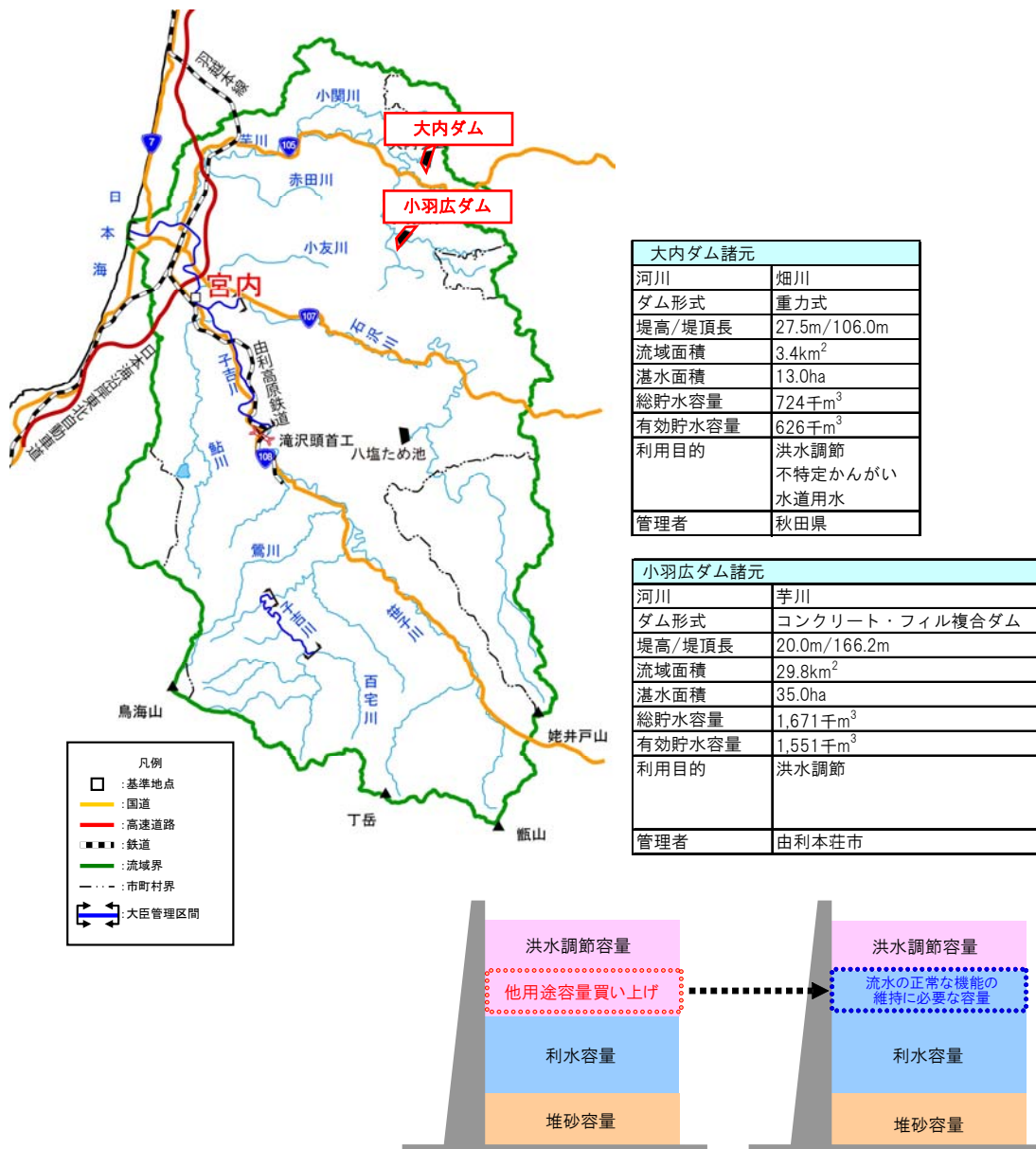
図 4.4-7 ダム容量買い上げのイメージ
