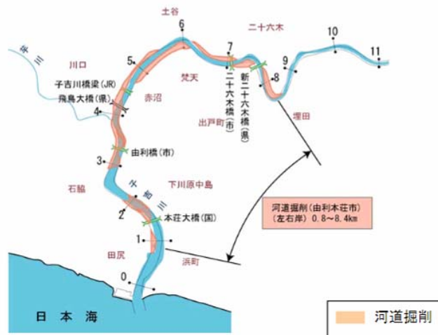
図 2.4-7 河道掘削位置図
