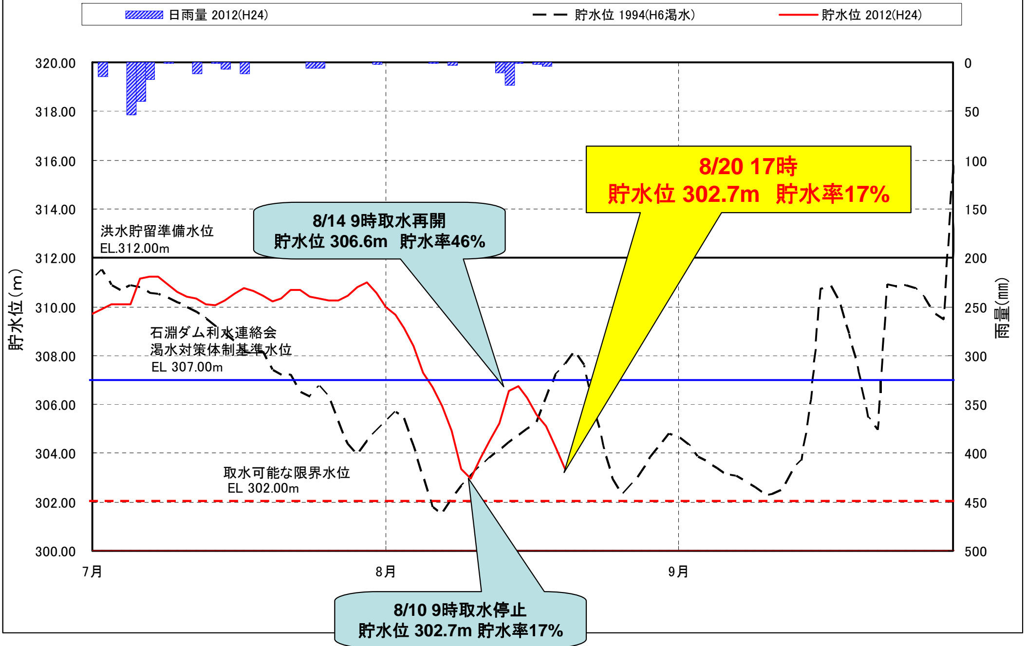
石淵ダム貯水位曲線
