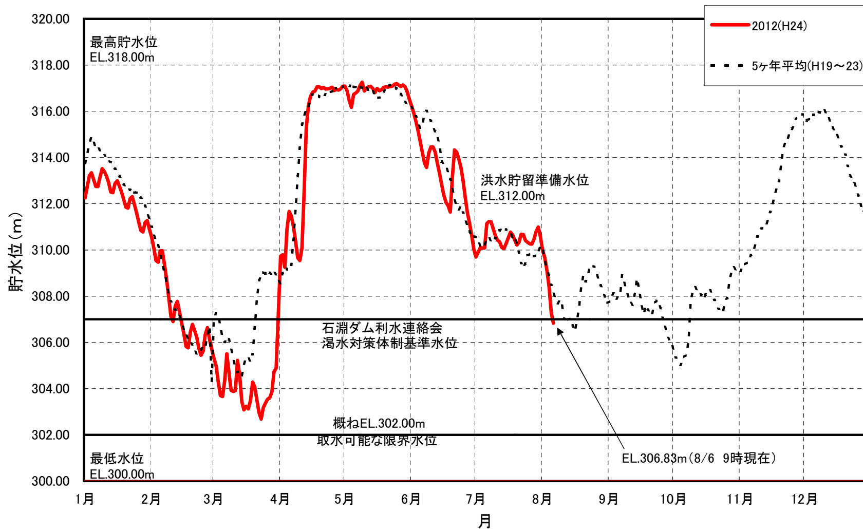
石淵ダム貯水位曲線 (8月6日9時現在)
