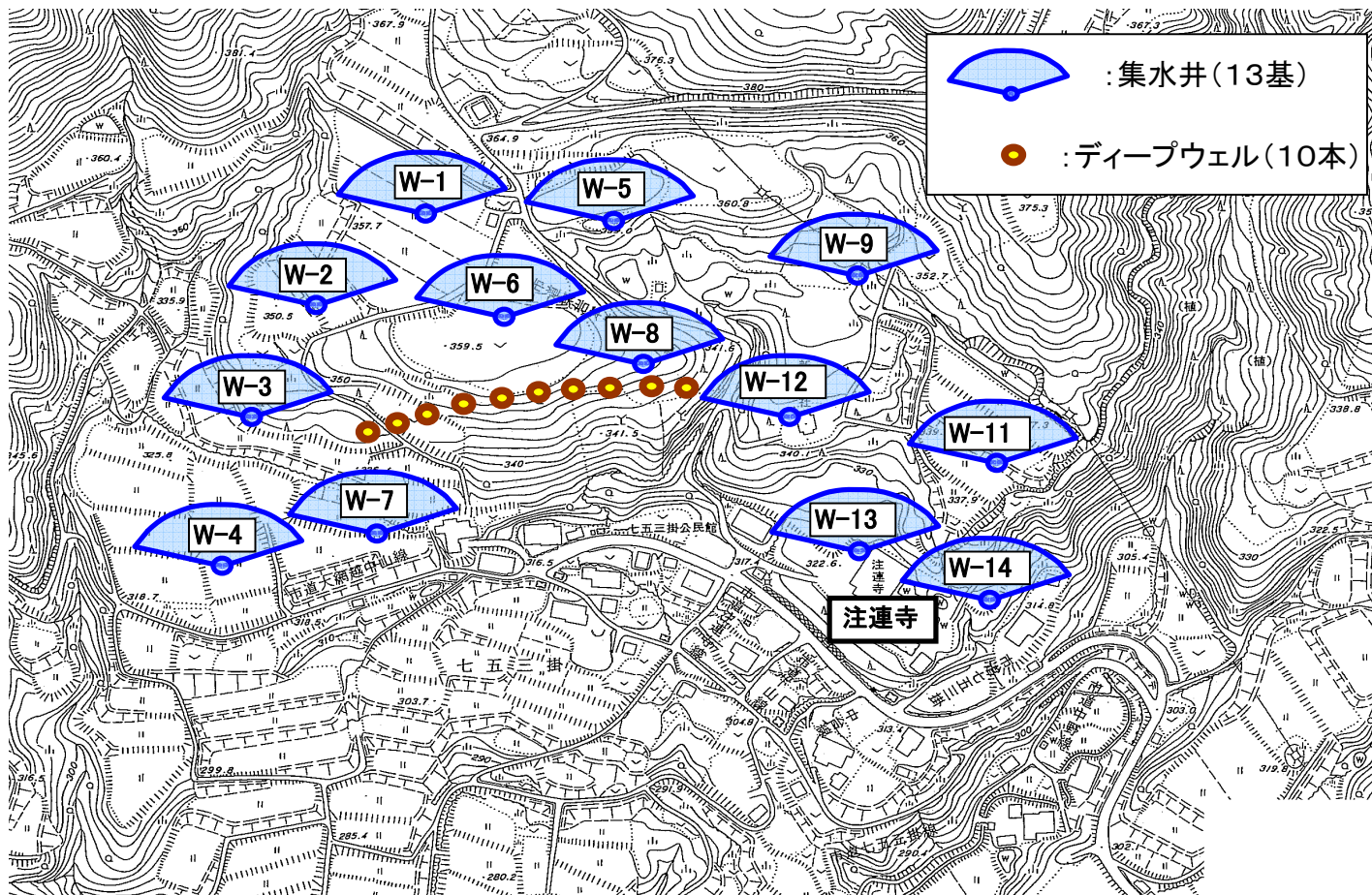
集水井工事進捗状況(7月29日現在)
