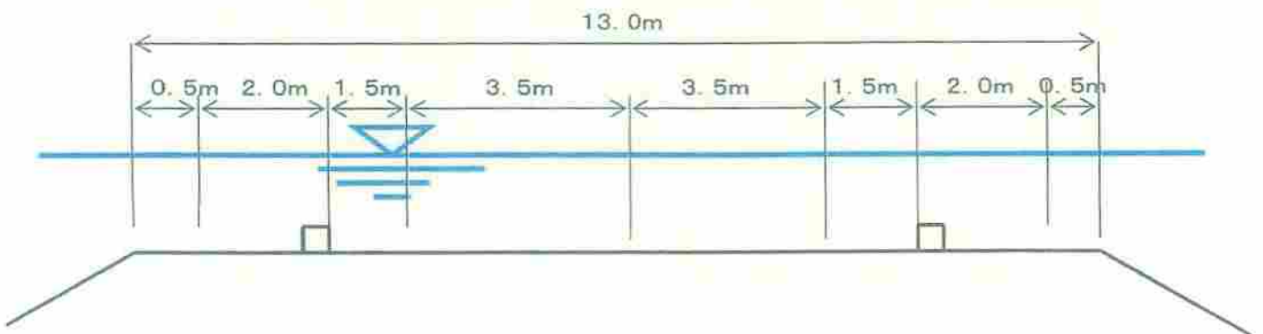
横断図
