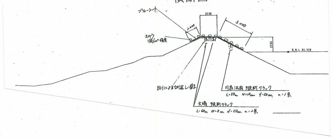
横断図
