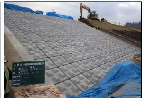
復旧工施工状況
