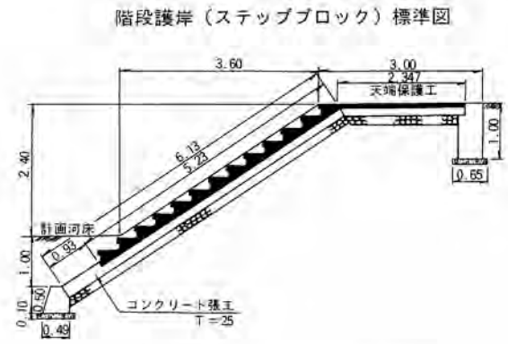
図 7-2 階段護岸標準図
