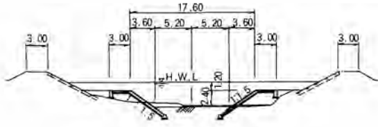
図 7-1 計画標準断面図
